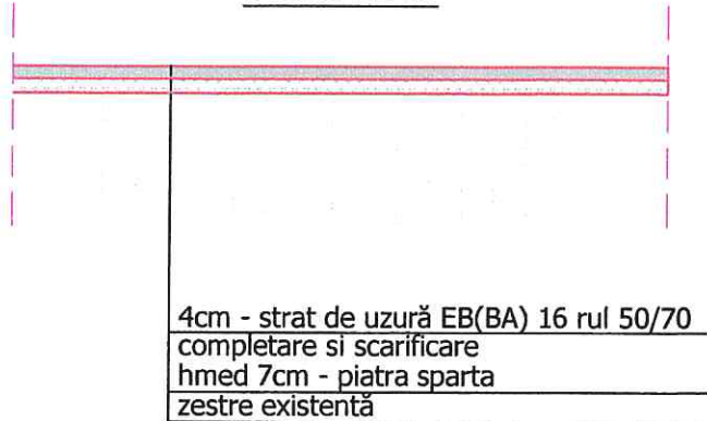
Detaliu de executie curte SRC1 scara 1:40
